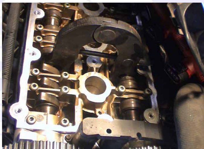
NOCKENWELLENFIXIERUNG
