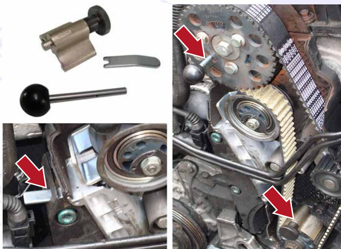
ARRETIERWERKZEUG
