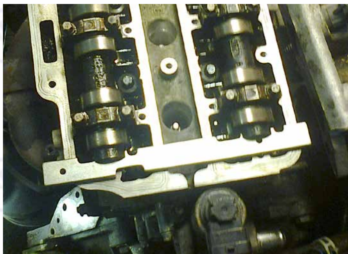
NOCKENWELLENLINEAL
