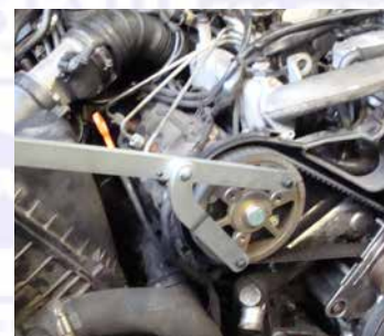
NOCKENWELLENRAD GEGENHALTER
