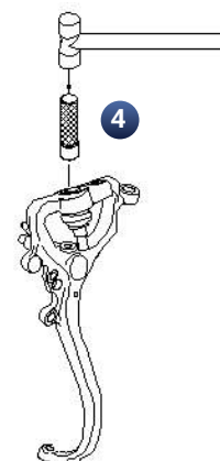
Ausbau des alten Kugelgelenks bei W220
