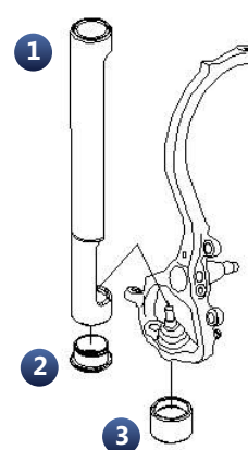
Einpressen des Kugelgelenks bei W220
