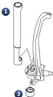
Einpressen des Kugelgelenks bei W123, W126
