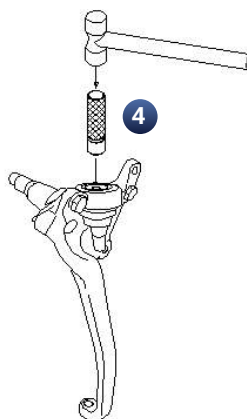
Ausbau des alten Kugelgelenks bei W123, W126
