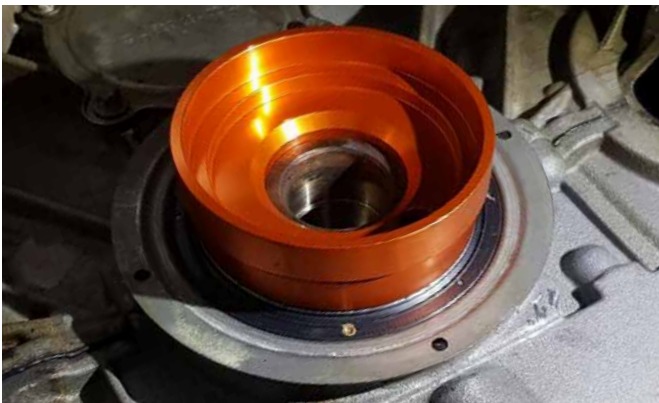
WELLENDICHTRING EINZIEHEN
