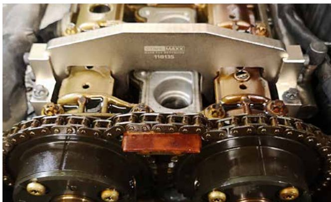
ARRETIERWERKZEUG FÜR NOCKENWELLEN 118135
