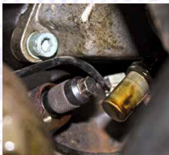
KURBELWELLEN ARRETIERUNG
