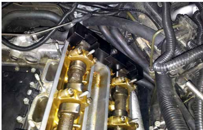
NOCKENWELLENFIXIERUNG
