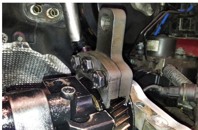
KLEMMVORRICHTUNG NOCKENWELLENRAD
