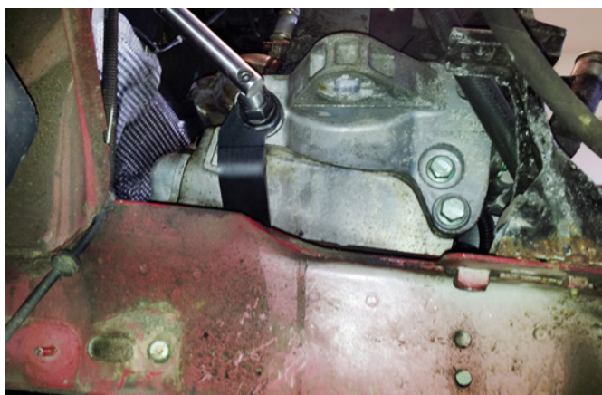
KURBELWELLENFIXIERUNG
