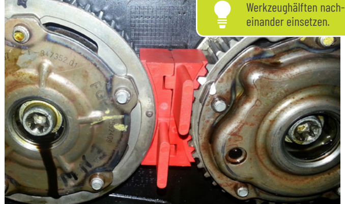
HALTEWERKZEUG FÜR NOCKENWELLENRÄDER 21030
