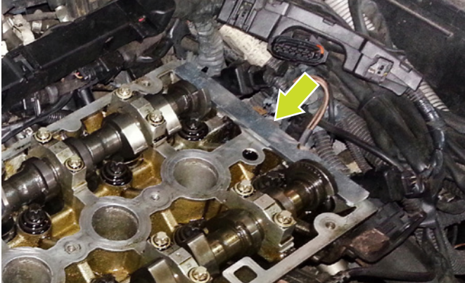
BEFESTIGUNGSWERKZEUG FÜR NOCKENWELLE KT11059
