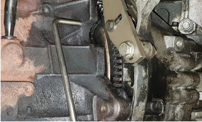
SCHWUNGRADARRETIERUNG, KURBELWELLENFIXIERUNG
