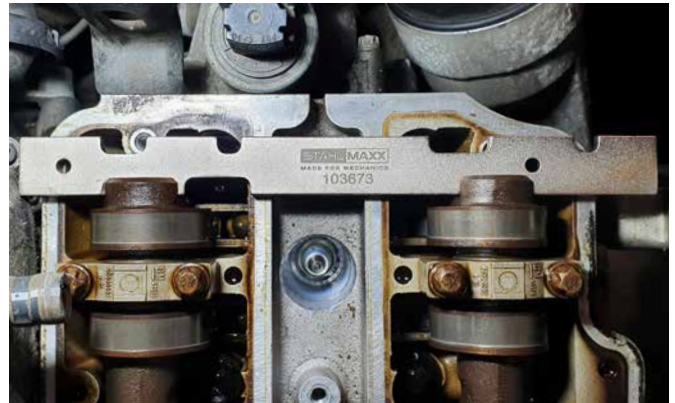
NOCKENWELLENLINEAL 103673
