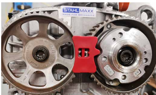
MONTAGEWERKZEUG FÜR NOCKENWELLE 112890
