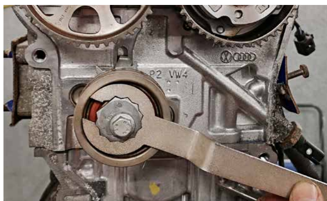
SCHLÜSSEL SW 30 FÜR ZAHNRIEMENSPANNER 112892
