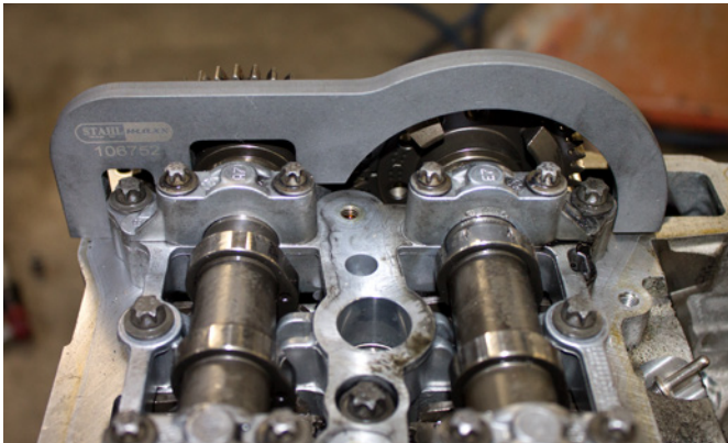
LEHRE ZUM FIXIEREN DER NOCKENWELLE 106752
