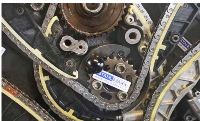
FIXIERDORN EINSPRITZPUMPE & NOCKENWELLE
