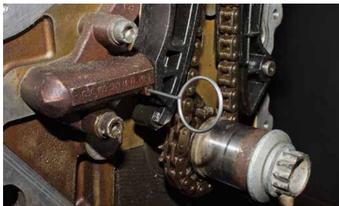
ARRETIERSTIFT FÜR KETTENSANNER 112906
