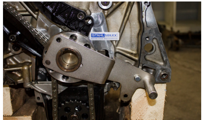
ABSTECKVORRICHTUNG FÜR KURBELWELLE 114192
