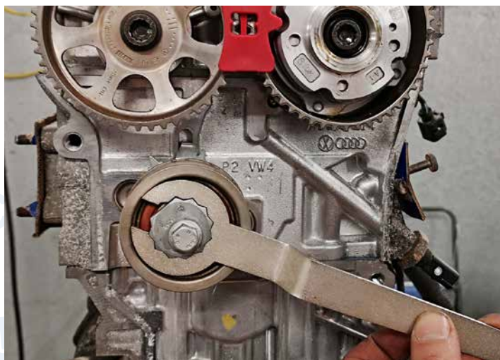
RINGSCHLÜSSEL FÜR ZAHNRIEMENSANNER
