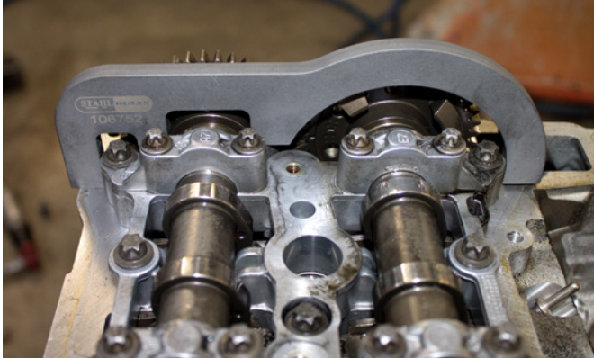
NOCKENWELLENARRETIERUNG
