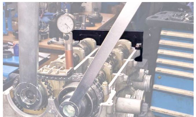
EINSTELLVORRICHTUNG 117468 MIT HALTEFEDERN 117469
