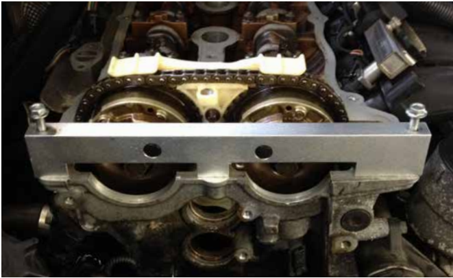
EINSTELLWERKZEUG FÜR VANOS-SENSOR 121117
