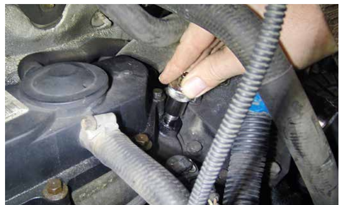
NOCKENWELLEN FIXIERWERKZEUG 103738
