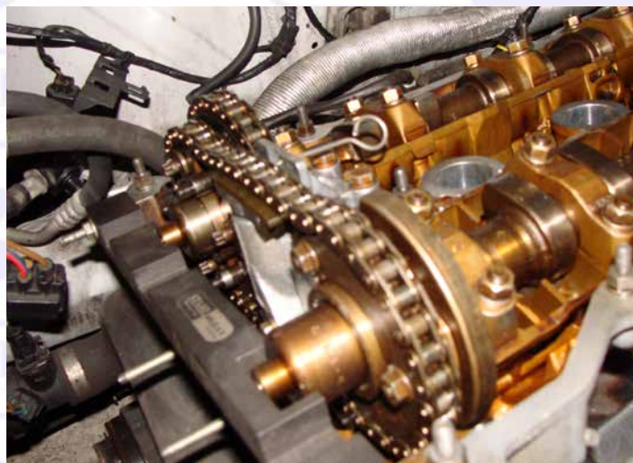
NOCKENWELLENFIXIERUNG - DETAIL
