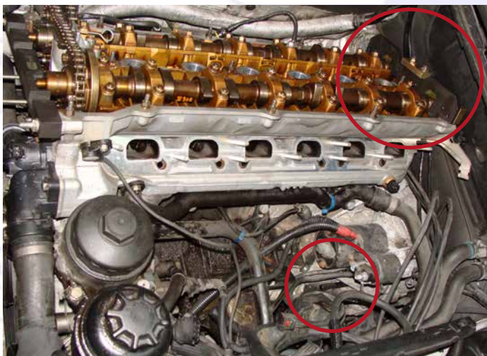
NOCKENWELLENFIXIERUNG, ABSTECKDORN
