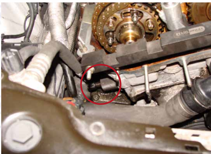
KETTENSPIANNER
